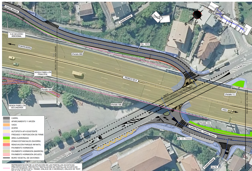
Reordenación de las intersecciones de Camiño Mouriño y Camiño da Igrexa con la carretera N-552 en el entorno del PK 150+500 de la AP-9.
